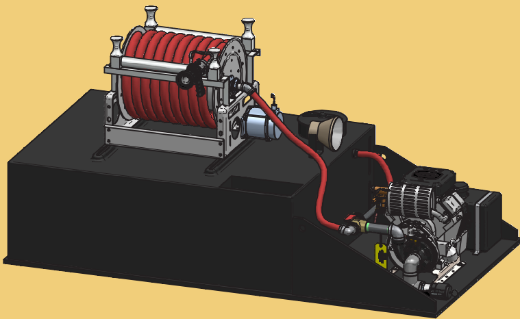
200 GALLON SKID SHOWN
