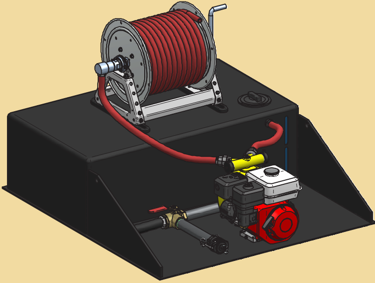
75 GALLON SKID SHOWN
